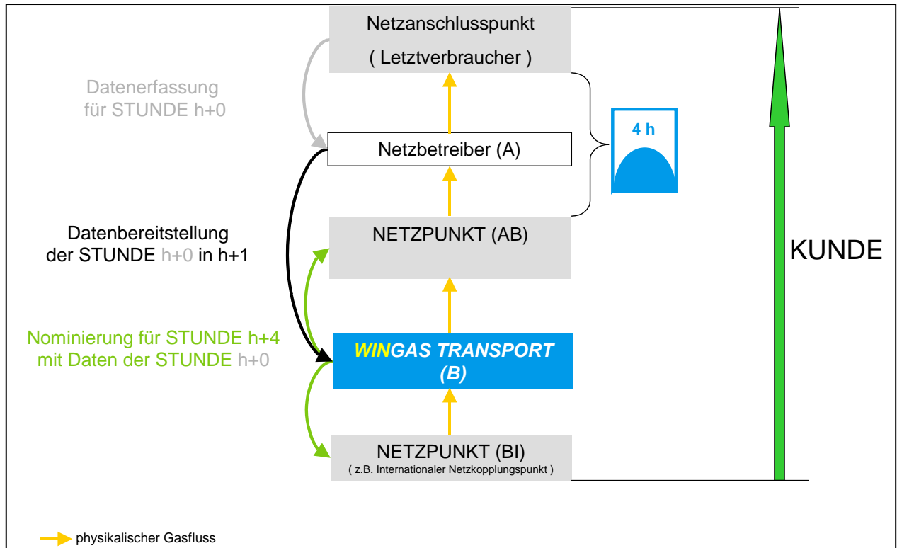
Bild: ZEITVERSATZVERFAHREN III (ohne BILANZAUSGLEICH durch WINGAS TRANSPORT)
